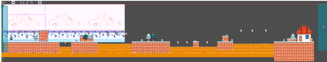
Figura 2 - TileSet Terreno
